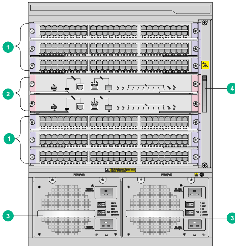
图1-4 S8600X-06-G-PoE 前面板示意图
