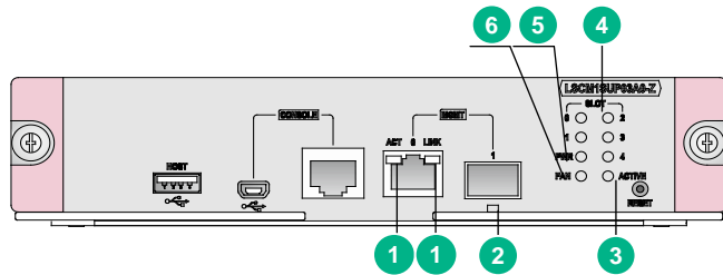
图1-1 LSCM1SUP03A0-Z 主控板指示灯示意图
