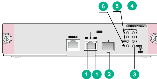
图1-2 LSCM3SUP03A0-ZE 主控板指示灯示意图
