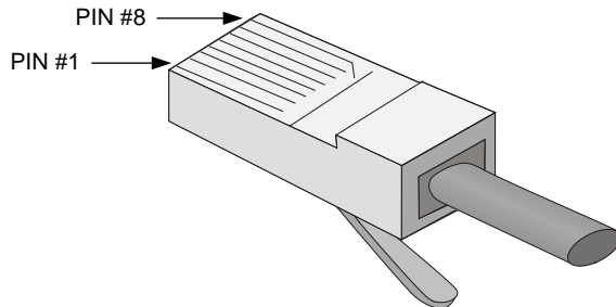
图1-1 RJ-45 连接器引脚序号示意图
