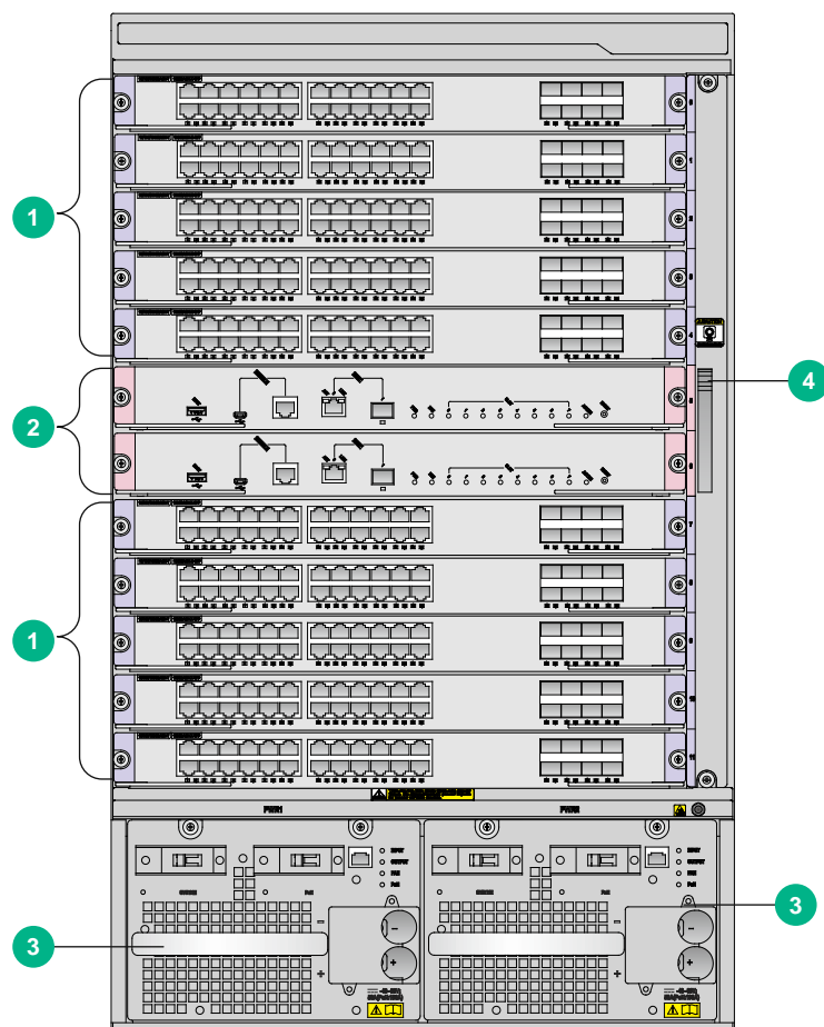
图1-5 S8600X-10-G 前面板示意图
