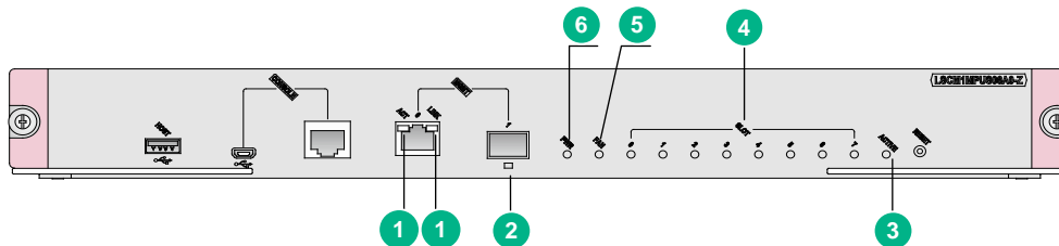
图1-3 LSCM1MPUS06A0-Z 主控板指示灯示意图
